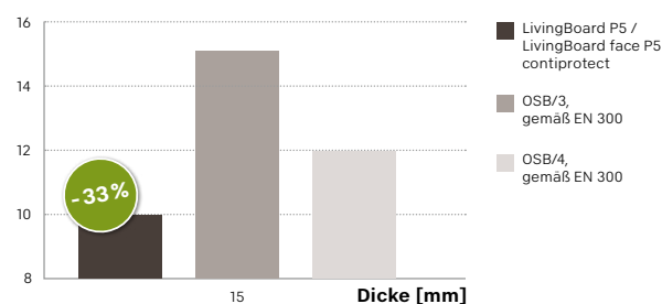
Dickenquellung in %
