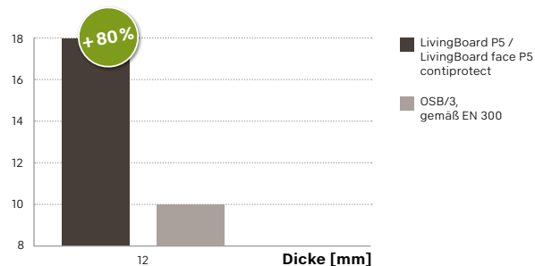
Biegefestigkeit quer zur Herstellrichtung in N/mm 2
